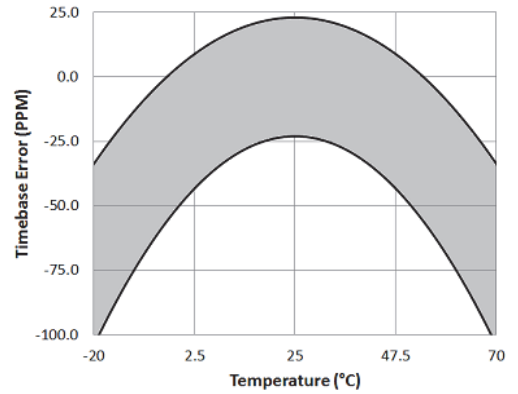
Schéma C : Précision du temps
