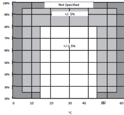
Schéma B : précision Humidité Relative
