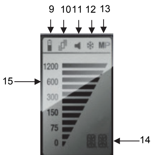
Fig. 12: Écran du détecteur des fuites de gaz
